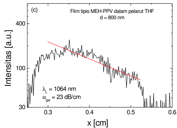
Gambar 7. Hasil pengukuran waveguide loss pandu gelombang planar MEH-PPV yang dibuat dengan pelarut kloroform, toluen dan THF pada panjang gelombang 1064 nm.
