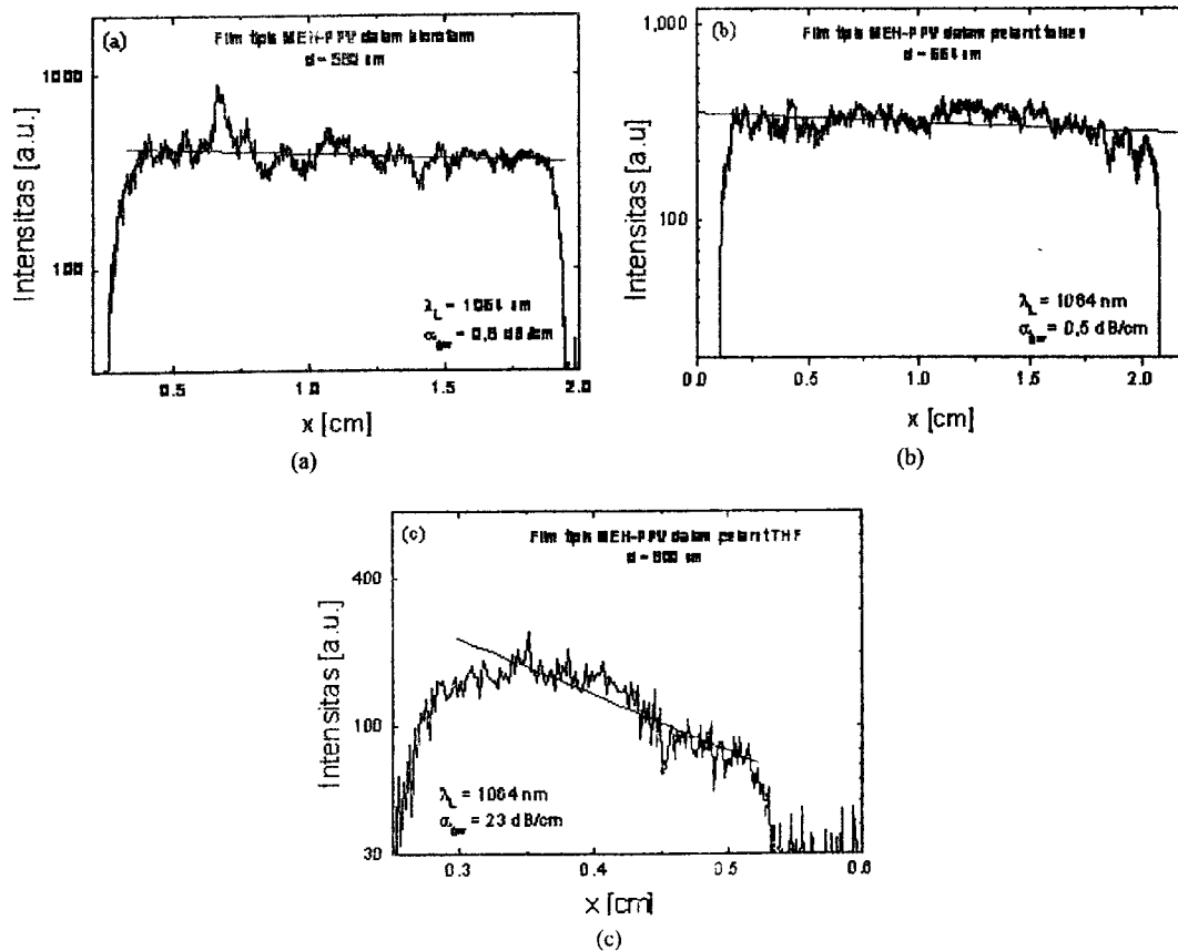
Gambar 7: Hasil pengukuran waveguide loss pandu gelombang planar MEH-PPV yang dibuat dengan pelarut kloroform, toluen dan THF pada panjang gelombang 1064 nm.
