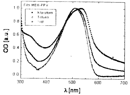
Gambar 5: Spektra UV-Vis film tipis MEH-PPV dengan pelarut kloroform, toluen, dan THF
