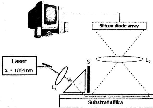
Gambar 3: Susunan eksperimen untuk pengukuran waveguide loss coefficient dari pandu gelombang planar.
