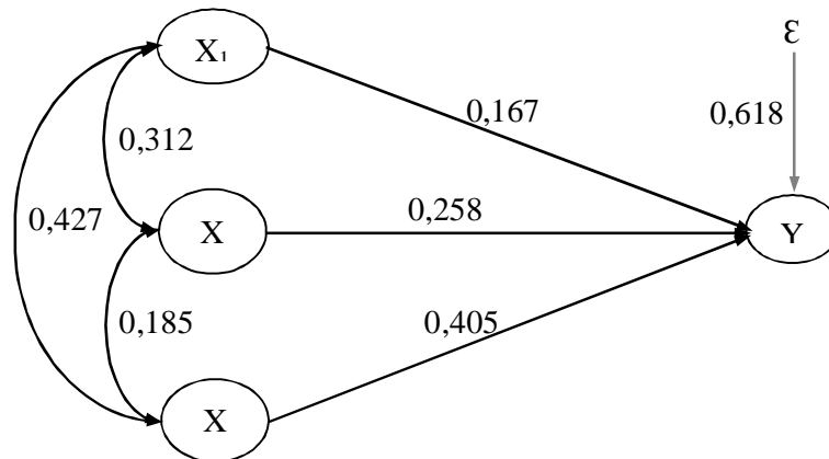
Gambar 4.2. Struktur hubungan antar variabel penelitian yang terbentuk.
