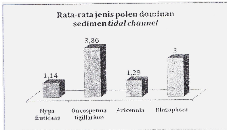
Gambar 5. Rata-rata jenis polen dominan pada sedimen tidal channel
