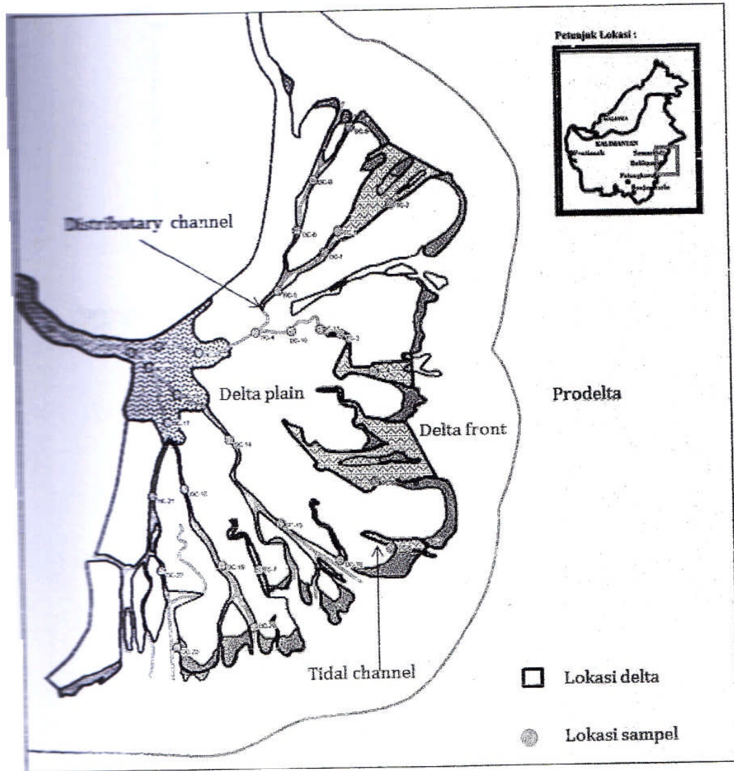
Gambar 1 .Lokasi daerah penelitian
