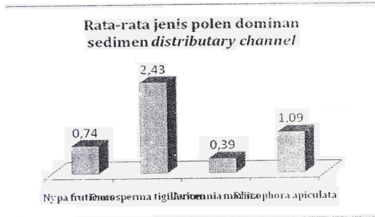
Gambar 4. Rata-rata jenis polen dominan pada sedimen distributary channel
