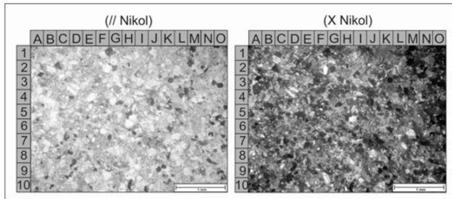
Gambar 5. Petrografi sayatan batupasir. O6= Kuarsa; F9= Piroksen; D3= Plagioklas; E8= Mineral Karbonat.
