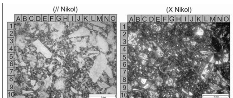
Gambar 9. Petrografi komponen breksi. O5= Mineral lempung, K2, J9= Kuarsa, M7, B9= Plagioklas, J7= Masa dasar.
