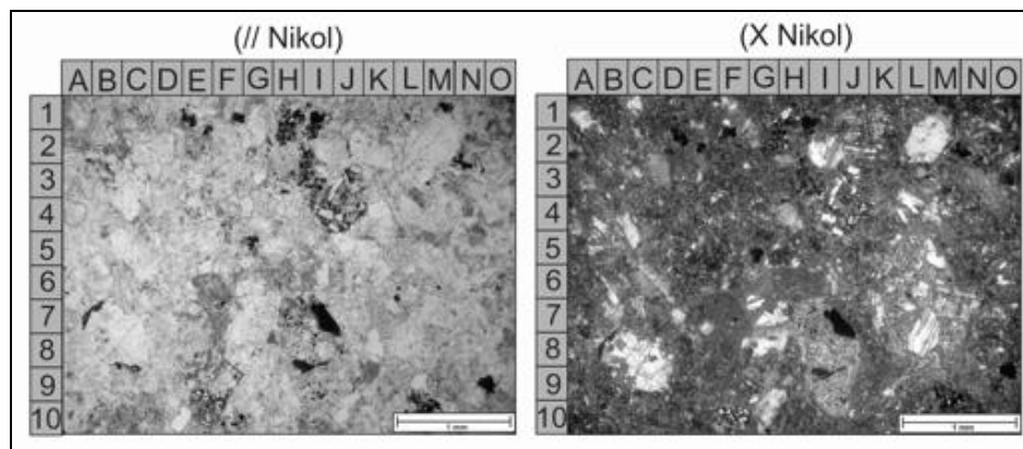
Gambar 8. Petrografi batupasir. I8,L6,J3= Fragmen batuan, H1= Kuarsa, L4,I2= Plagioklas.
