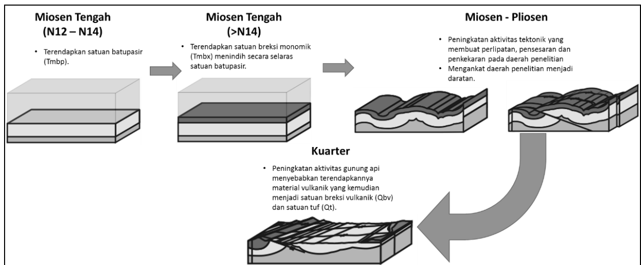
Gambar 14. Model Sejarah Geologi Daerah Penelitian
