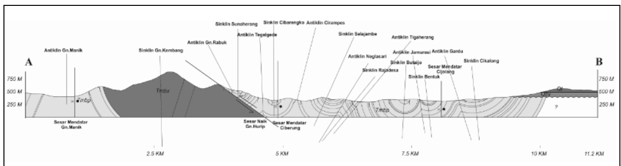
Gambar 3. Penampang Geologi Daerah Penelitian.
