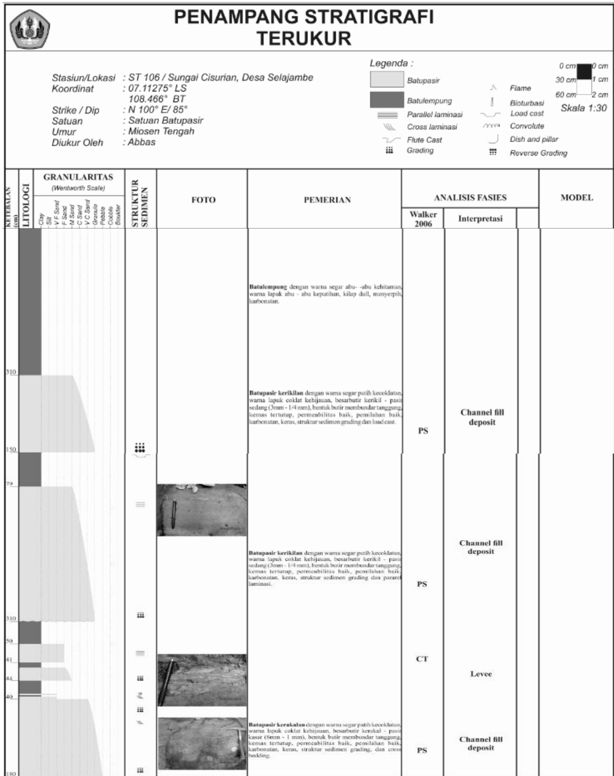
Gambar 6 (b). Penampang Stratigrafi Terukur Satuan batupasir.
