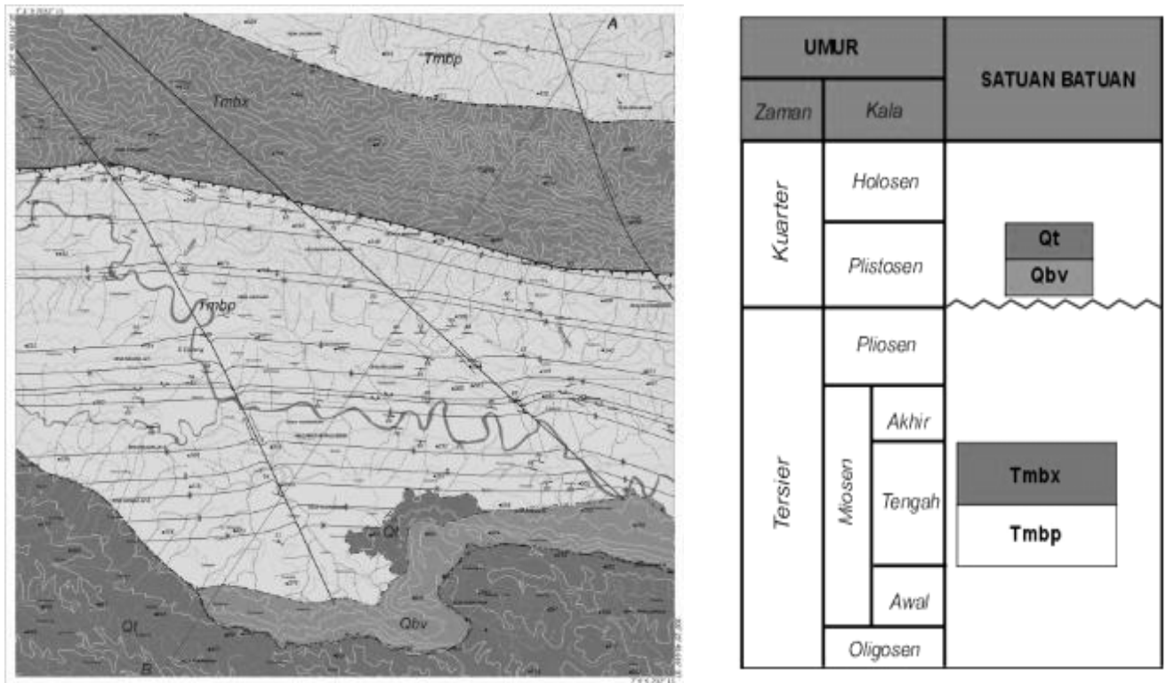
Gambar 2 (kiri). Peta Geologi Daerah Penelitian, dan Tabel 1 (kanan). Kolom Stratigrafi Daerah Penelitian
