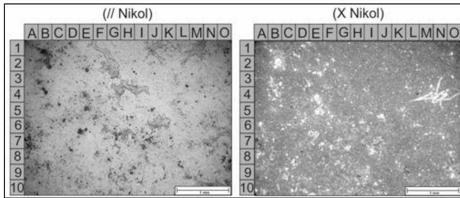
Gambar 13. Petrografi tuf. J5=Kuarsa, B1=Piroksen, J3=Gelas.
