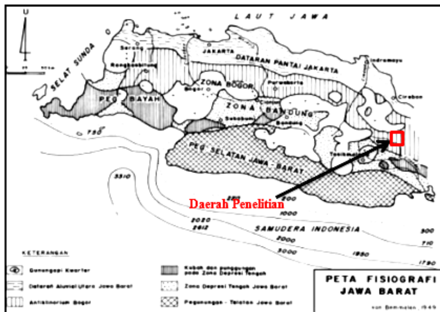
Gambar 1. Fisiografi Regional Daerah Penelitian (Van Bemmelen dalam Martodjojo, 2003)
