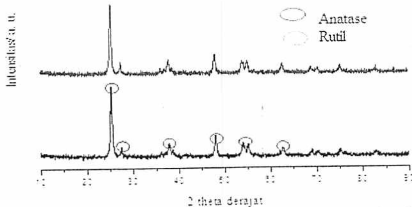
Gambar 5. Pola difraksi hasil karakterisasi dengan XRD dari titanium(IV) oksida Degussa P25, titanium(IV) oksida-platina 0,5%, dan titanium(IV) oksida-platina 1%.
