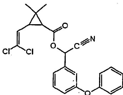
Gambar 6. Struktur kimia sipermetrin
