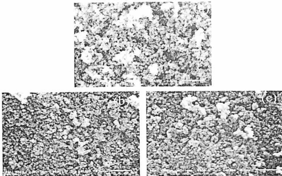
Gambar 2. Hasil karakterisasi SEM : (a) titanium(IV) oksida, (b) titanium(IV) oksida-platina 0,5%, dan (c) titanium(IV) oksida-platina 1%.
