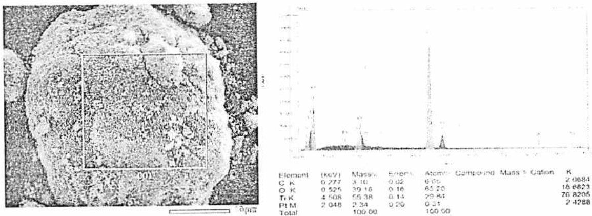
Gambar 4. Hasil karakterisasi SEM-EDX titanium(IV) oksida-platina 1%.
