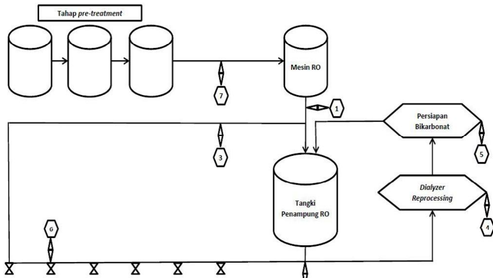
Gambar 1 Skema Unit Hemodialisis dan Lokasi Titik Pengambilan Sampel
